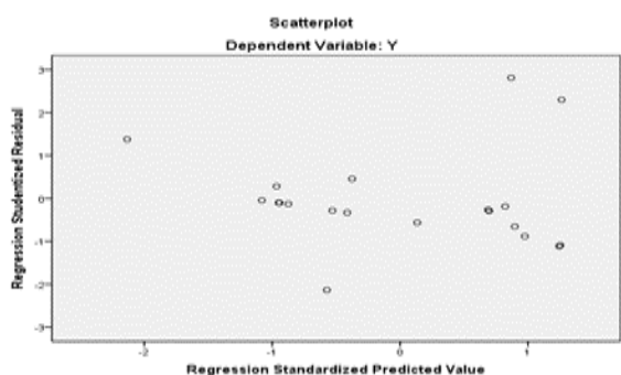
Gambar 2 Uji Heterokedastisitas
